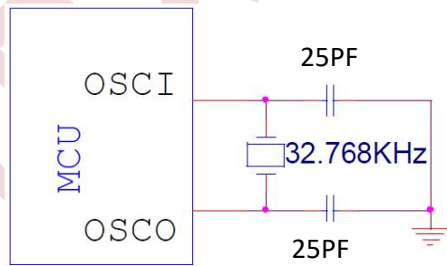
32.768KHz 参考典型电路图
