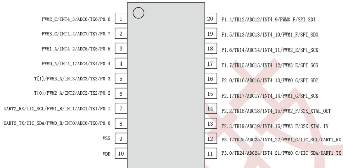
图 5-1-4 SOP20/TSSOP20 封装引脚图
