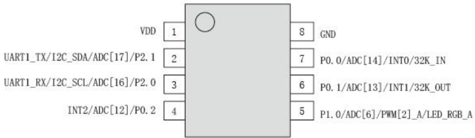
图 5-1-6 SOP8 封装引脚图
