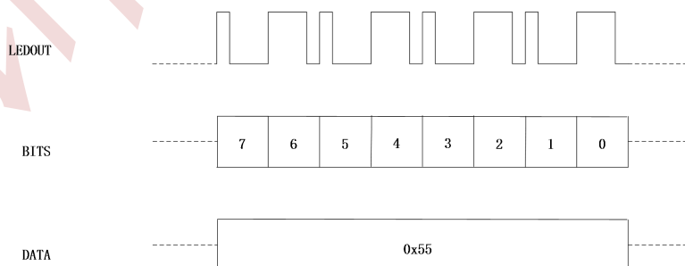
图 18-2-3 级联 LED 时序图
