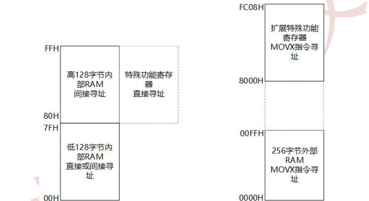
图 7-1-1 RAM 组织结构图
