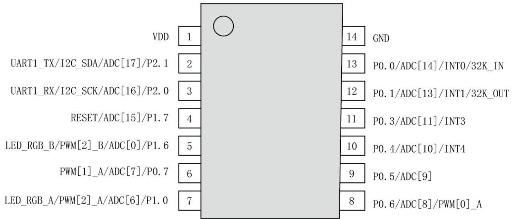
图 5-1-3 SOP14 封装引脚图
