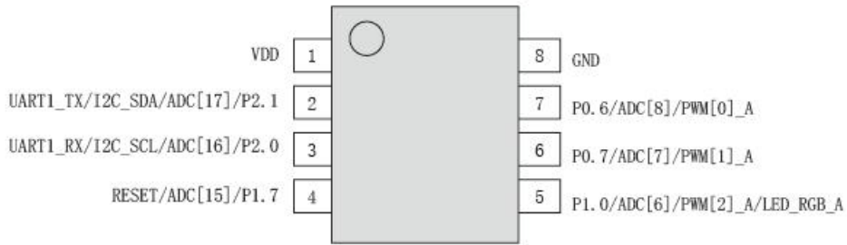
图 5-1-5 SOP8 封装引脚图
