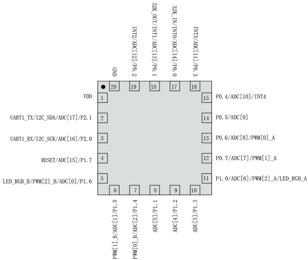
图 5-1-4 QFN20 封装引脚图
