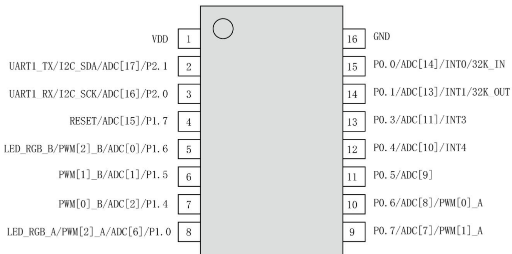
图 5-1-2 SOP16 封装引脚图
