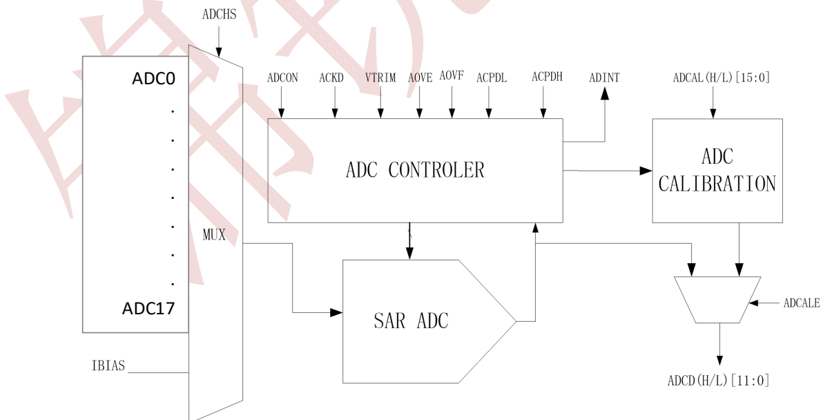
图 19-3-1 ADC 结构示意图
