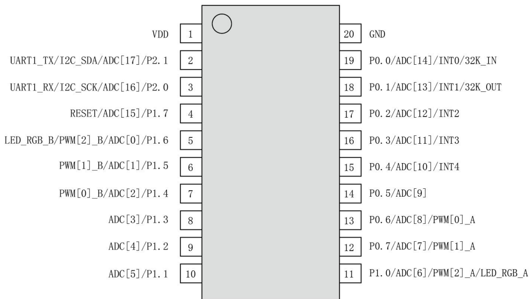
图 5-1-1 TSSOP20/SOP20 封装引脚图
