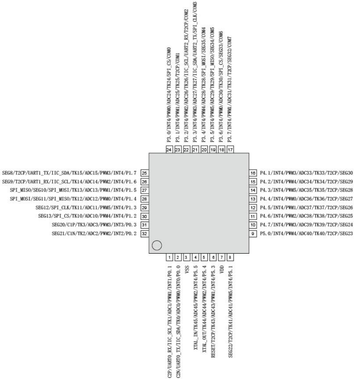
图 5-1-3 LQFP32 封装引脚图
