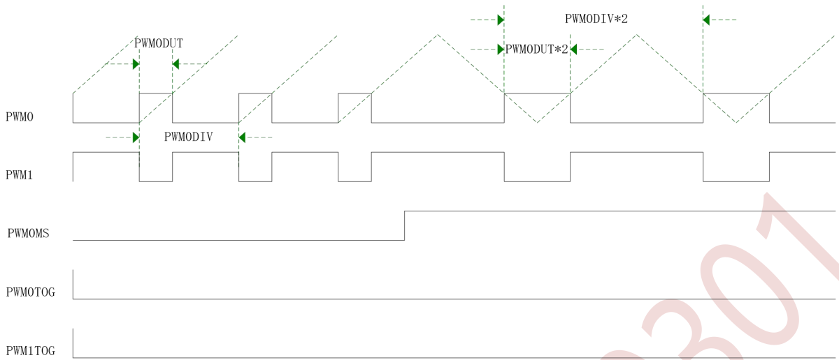
图 18-2-4 PWMTOG=0 时 PWM0、PWM1 输出互补波形
