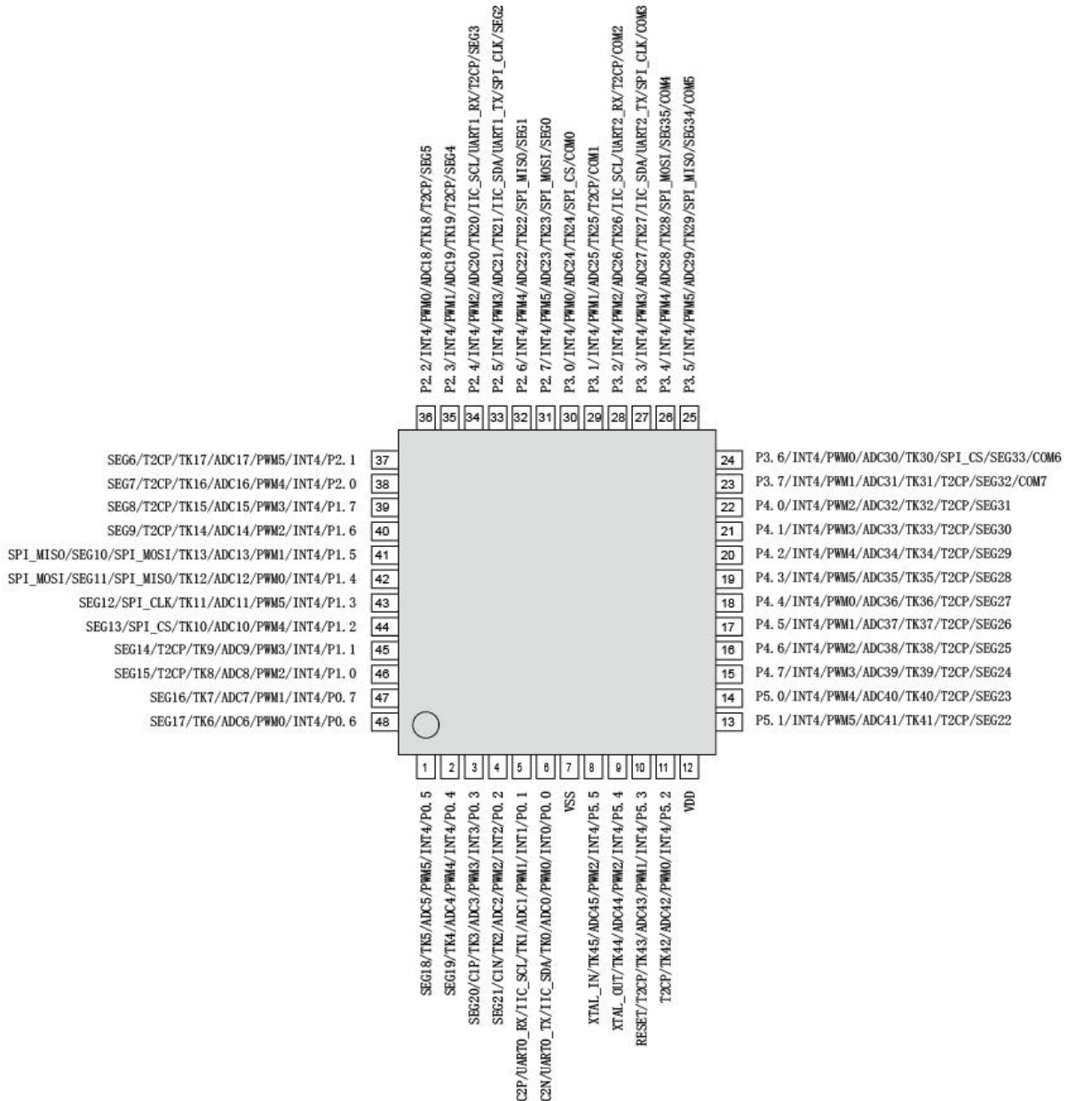
图 5-1-1 LQFP48 封装引脚图
