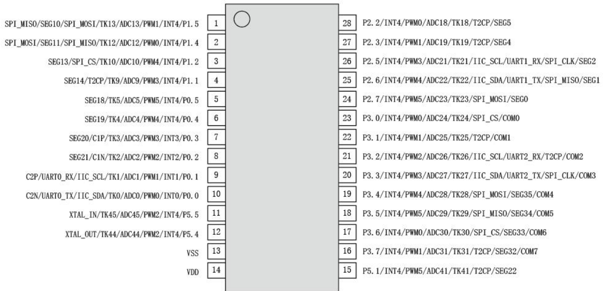
图 5-1-5 SOP28 封装引脚图
