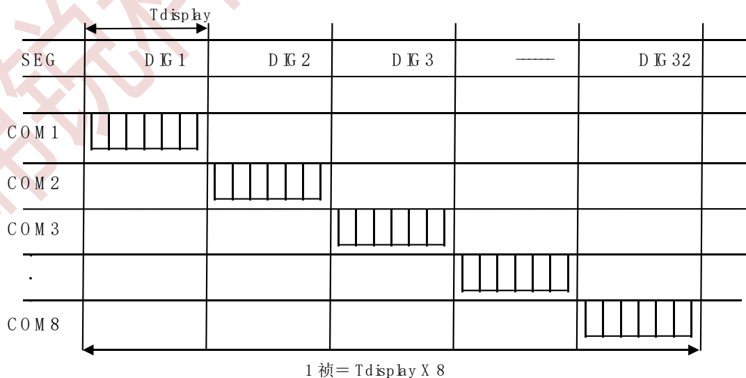
图 23-2-1-2 LED 驱动波形
