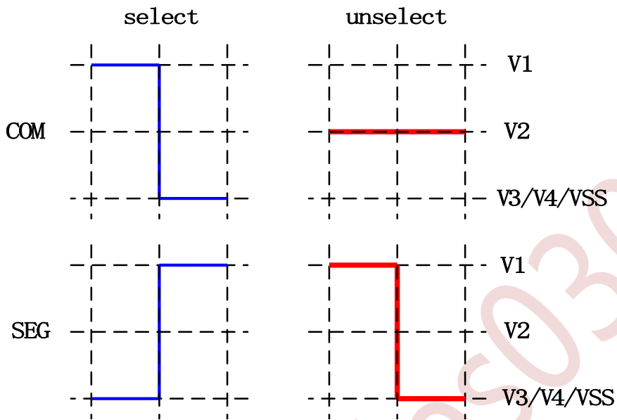
图 23-1-1-2 LCD 偏压比 1/2 信号
