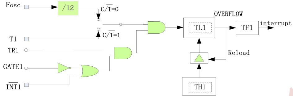
图 12-2-2 定时器 1 的模式 2
