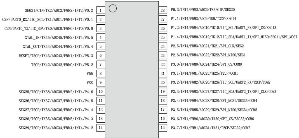
图 5-1-4 SOP28 封装引脚图
