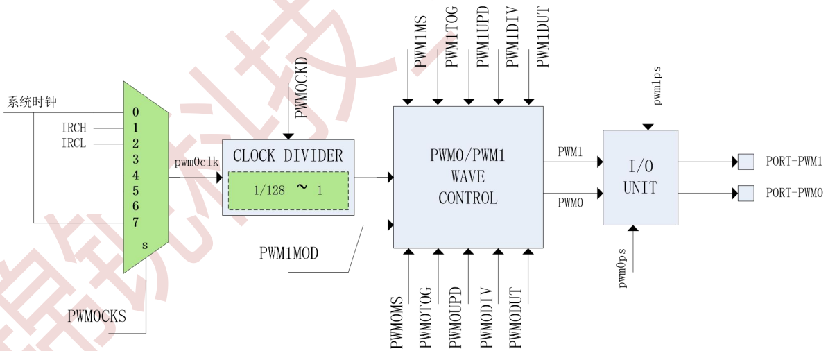
图 18-2-3 PWM0、PWM1 原理示意图
