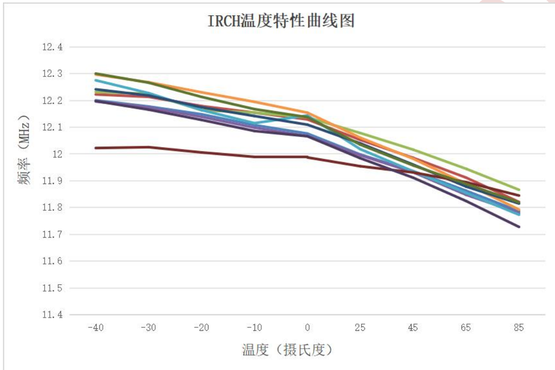
图 26-5-1 IRCH 温度特性曲线图
