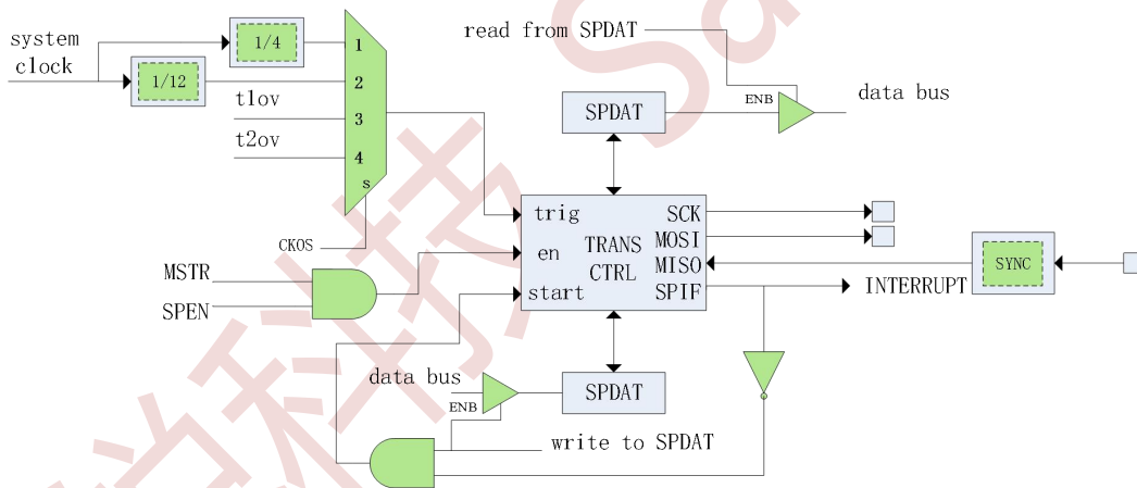
图 19-1-1 SPI 主机模式示意图
