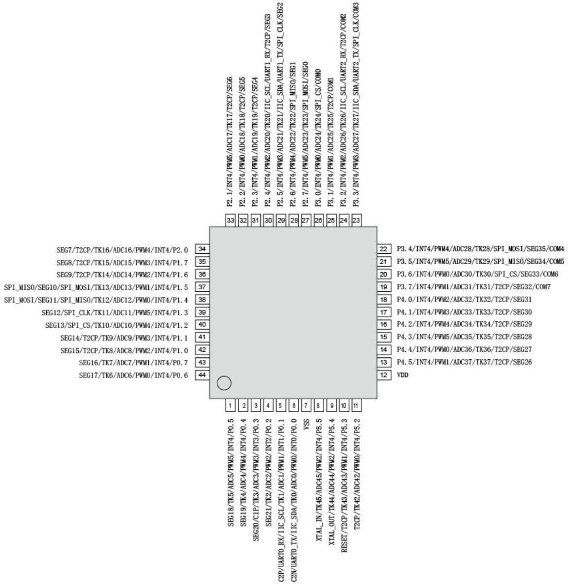
图 5-1-2 LQFP44 封装引脚图
