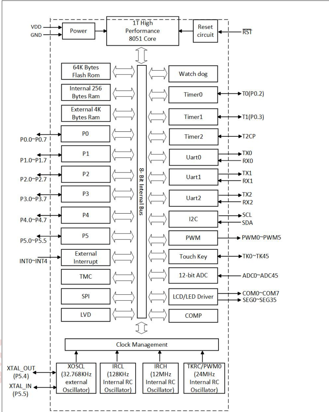
图 4-1 芯片框图
