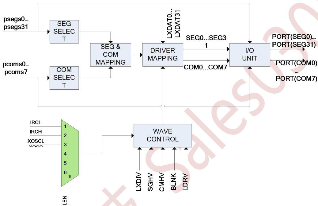
图 23-2-1-1 LED 原理示意图
