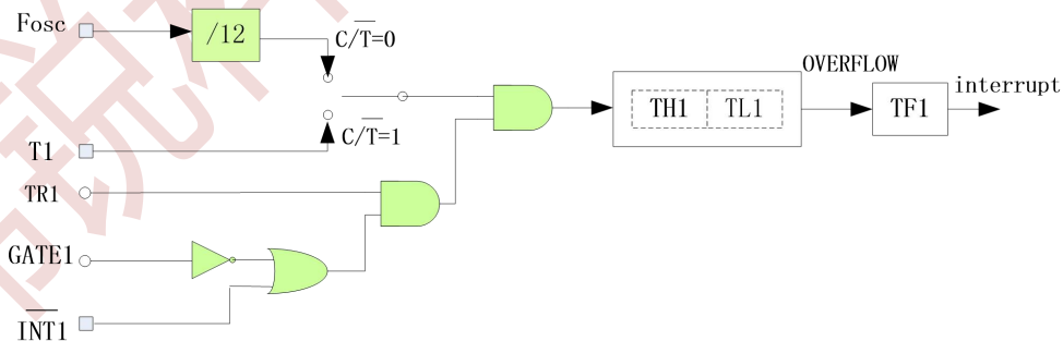
图 12-2-1 定时器 1 的模式 0 和 1
