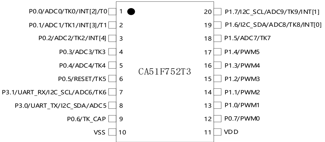
图 5-1-1 TSSOP20 封装图
